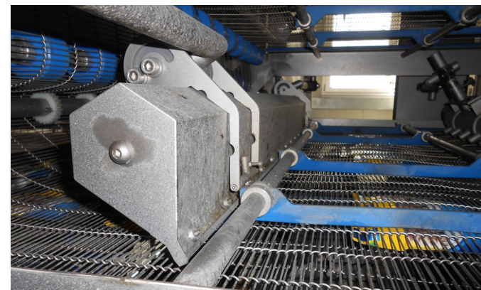
Beutelabbläsung .mit Niederhalteband
